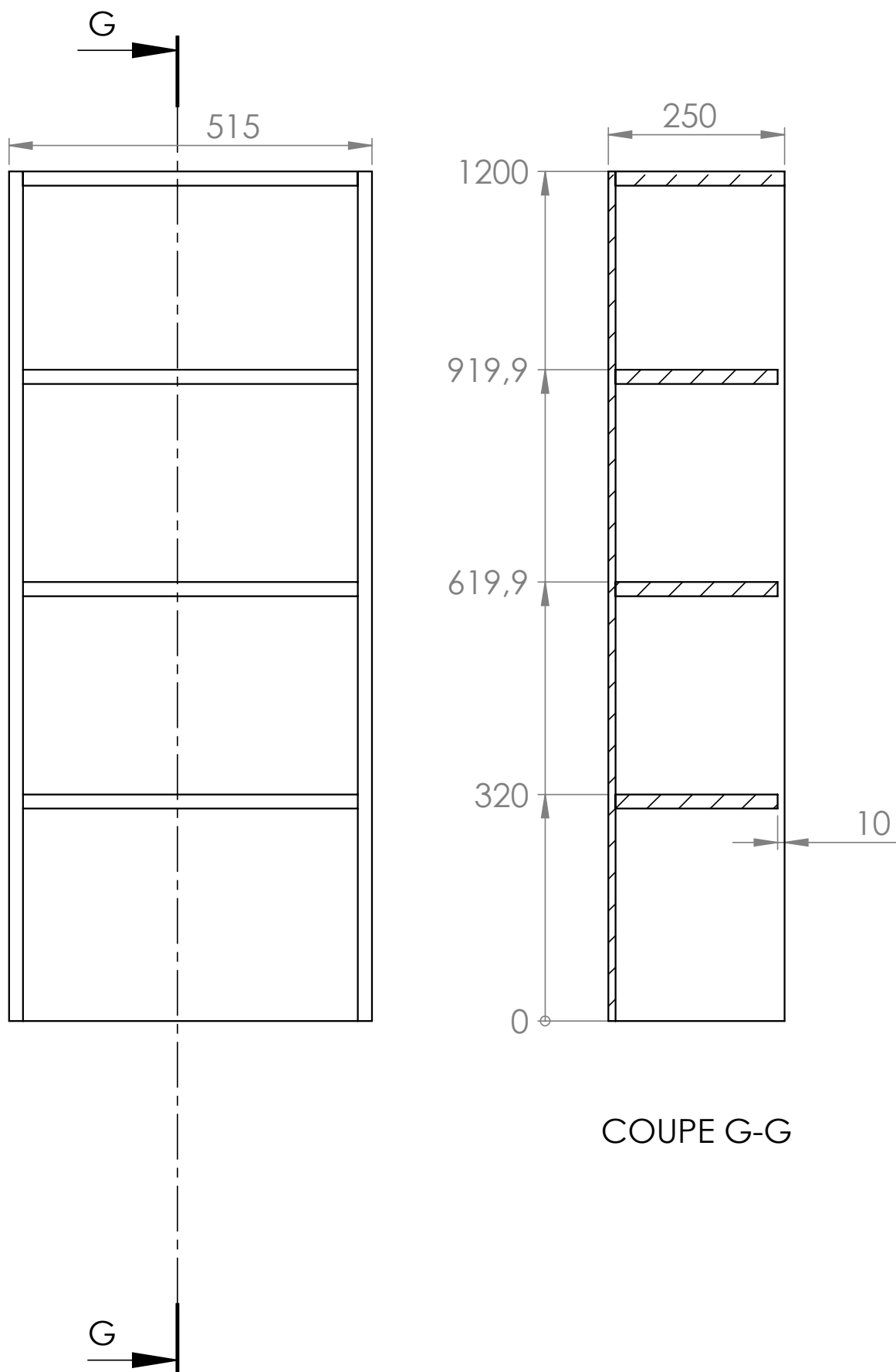
ANNEXE P Meuble C - Élévation et coupe
