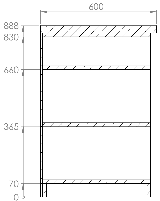
COUPE N-N
