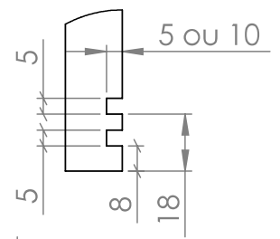
DÉTAIL A ECHELLE 1 : 2
