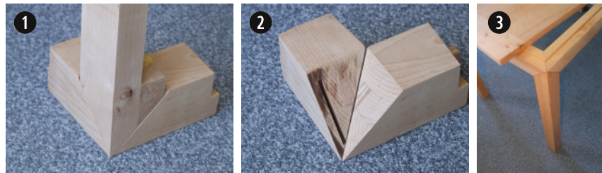
Détail de l'assemblage des pieds de la table.
