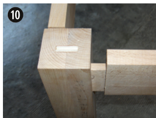
Un assemblage à tenon et mortaise.
