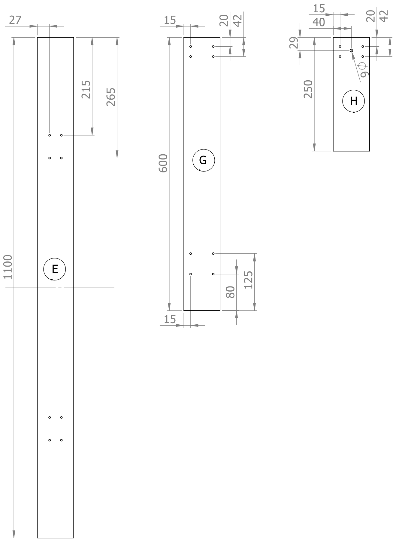
ANNEXE C Vues de détail des perçages
